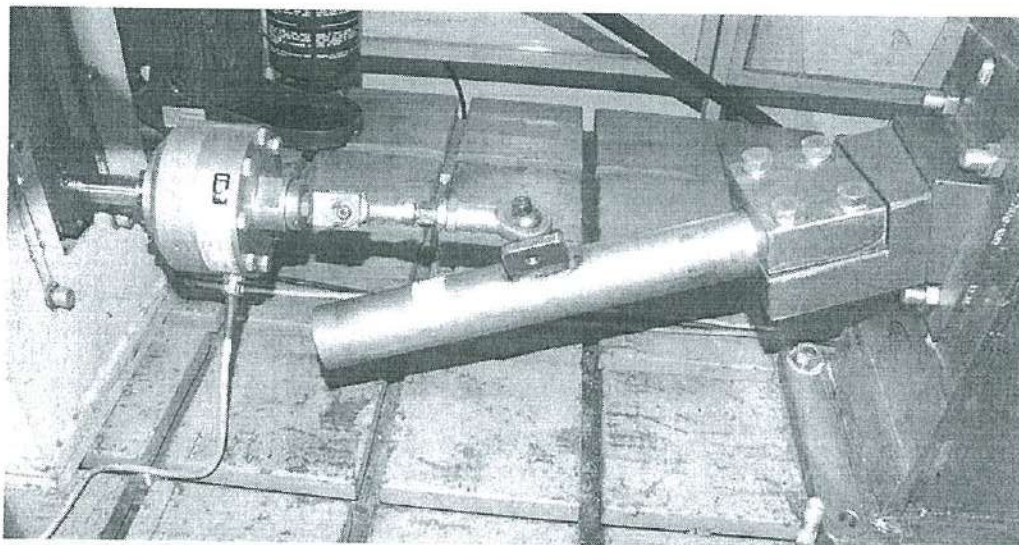
Рис 1. Схема испытания / Fig 1. Scheme of the test.
